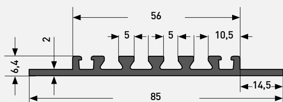
LMS 3319 | biegefähig, gelocht
