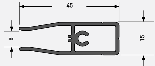
Einfassleiste 8 mm | LMS 4052
